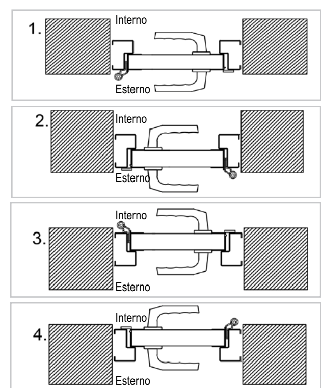
Opzioni di montaggio e senso di apertura delle porta laterali doppia anta.
